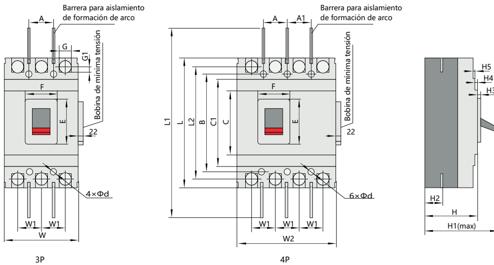
Dimensiones totales y de montaje del NM1-400, 630, 800, 1250 (tipo fijo)
