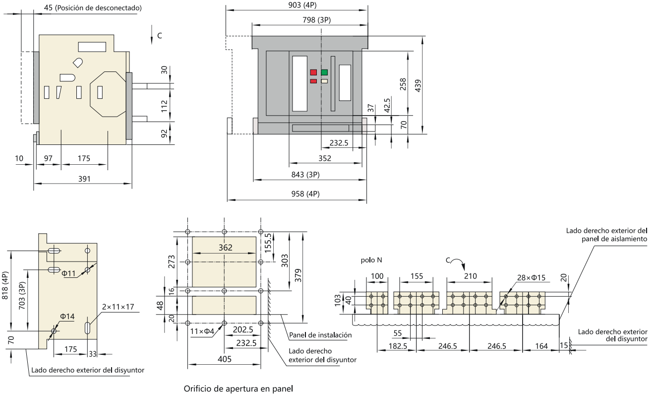
Orificio de apertura en panel
